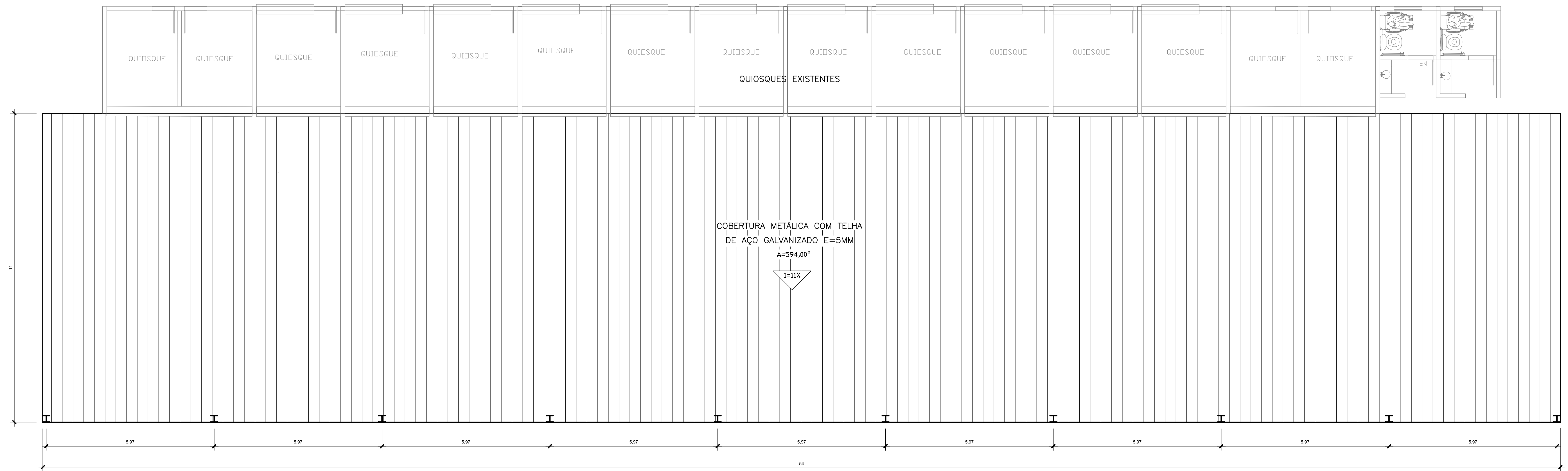
PLANTA BAIXA Escala 1/75
