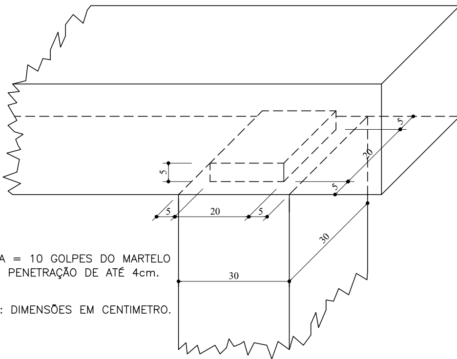
DETALHE DE ENCAIXE COM ESPIGA
