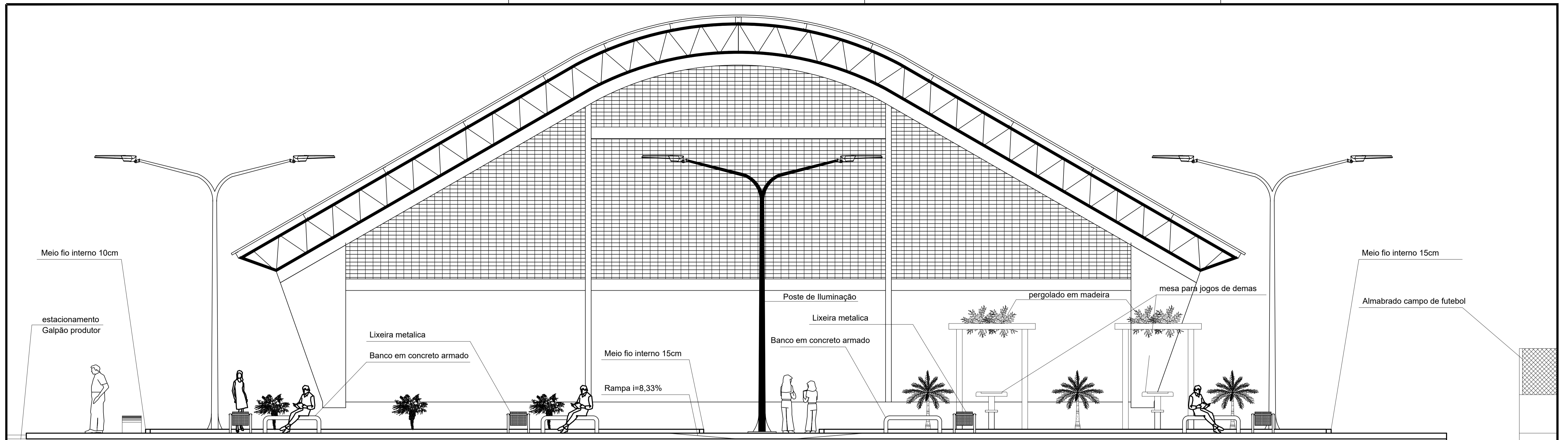
ELEVAÇÃO 01 Esc. 1:50
