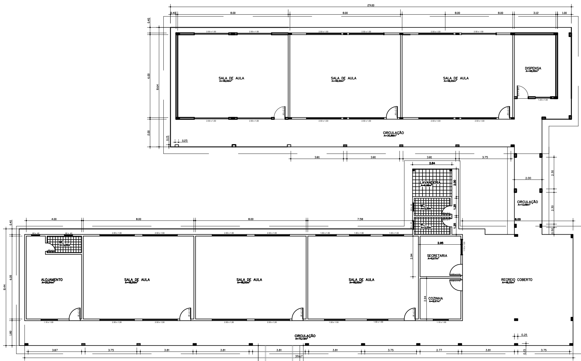
PLANTA BAIXA - ESCOLA NOSSA SENHORA APARECIDA Esc: 1/125
