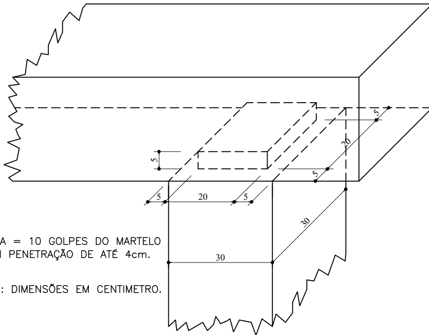
DETALHE DE ENCAIXE COM ESPIGA
