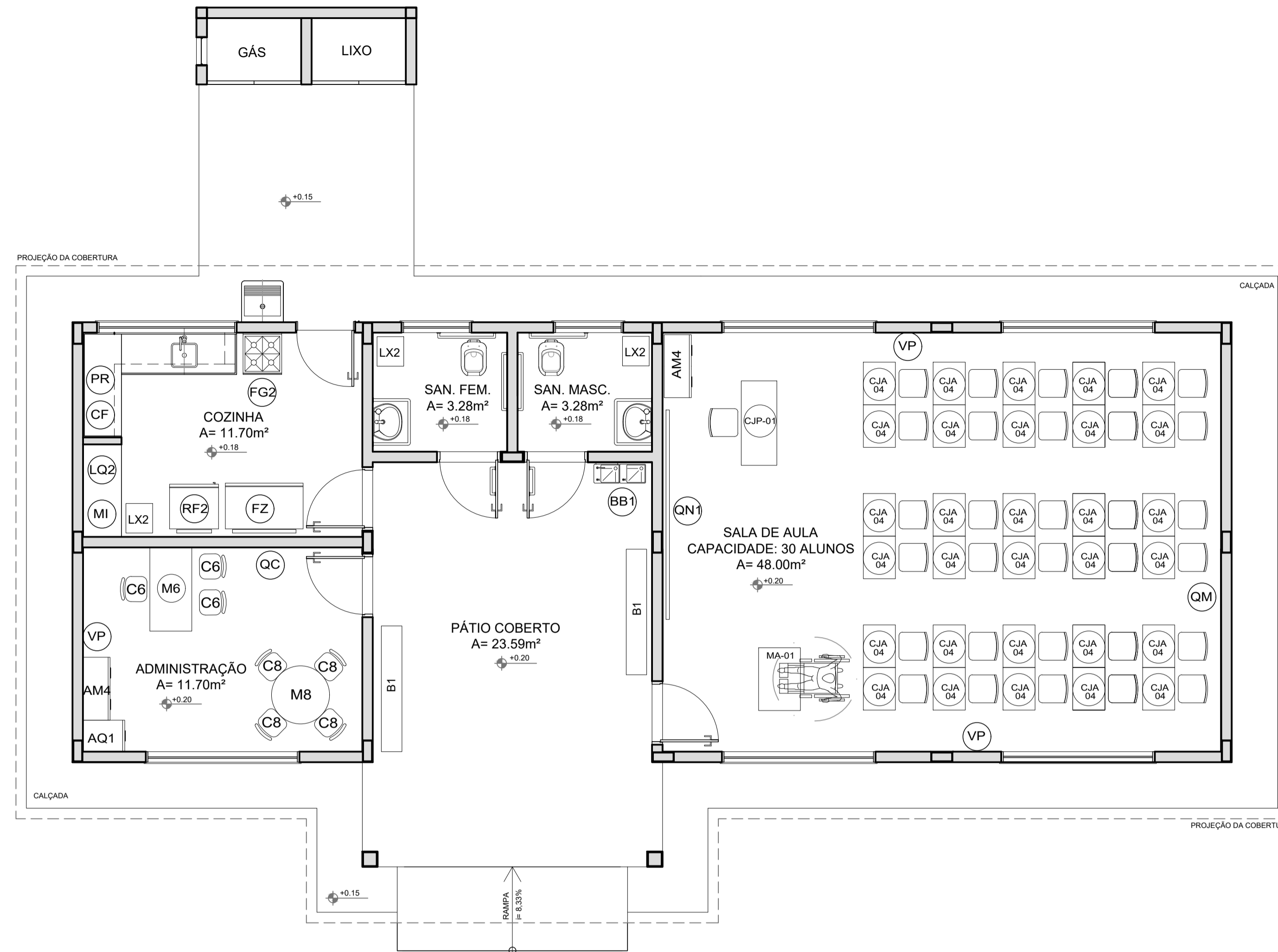
1 PLANTA BAIXA DE LEIAUTE ESCALA 1/50
