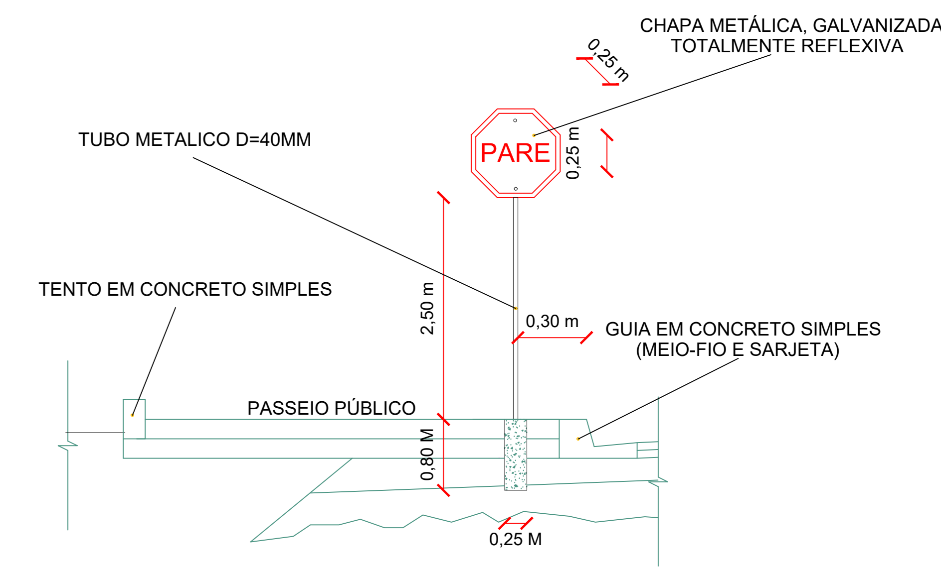
... DETALHE DA PLACA DE ... ... SINALIZAÇÃO VERTICAL - R-1 ... SEM ESCALA
