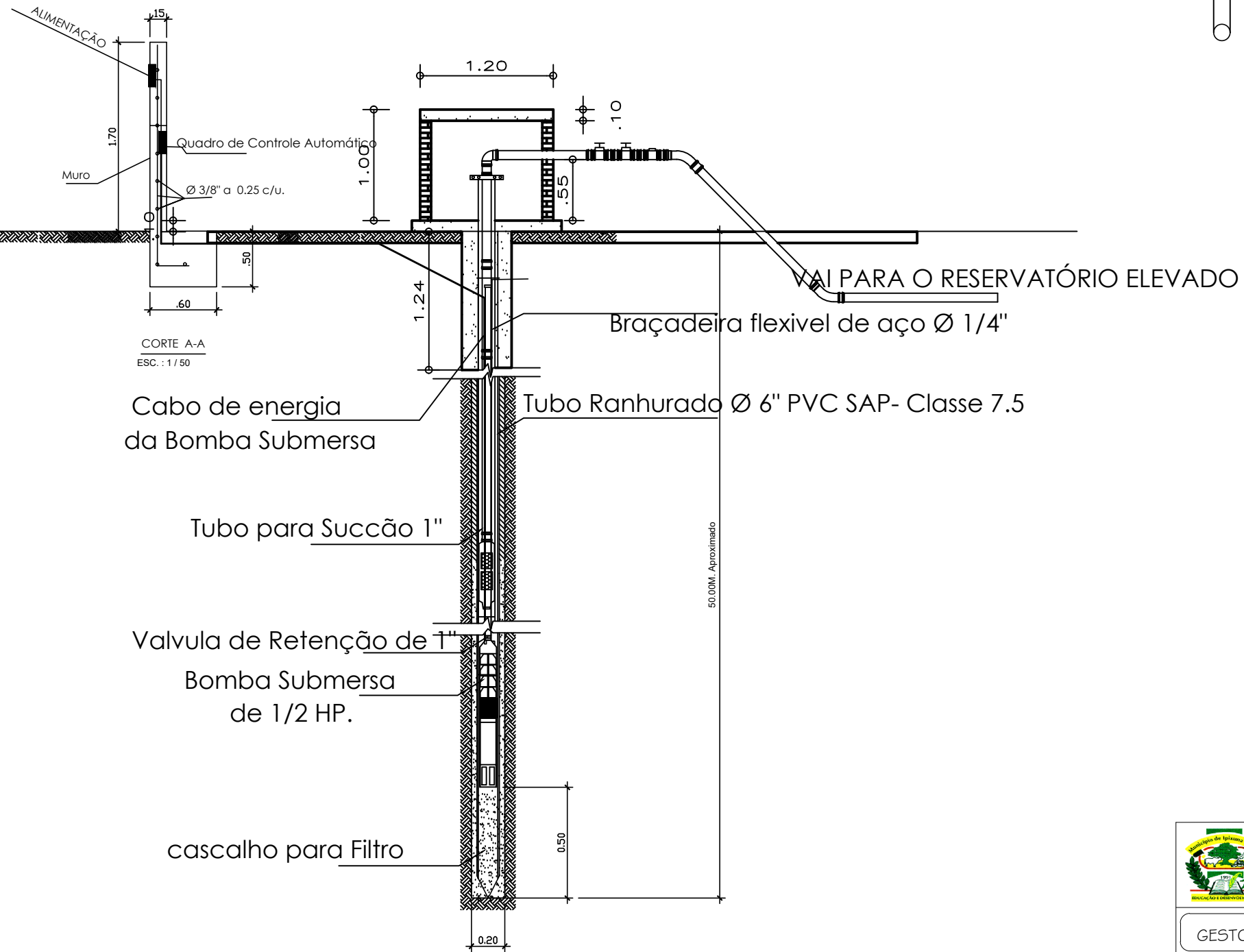
CORTE 1 - 1 DETALHE DE BOMBA SUBMERSA ESC.: 1/20
